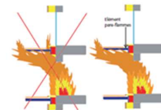
▲ Figure 26 - Pare-flammes entre structure rattachée et façade
