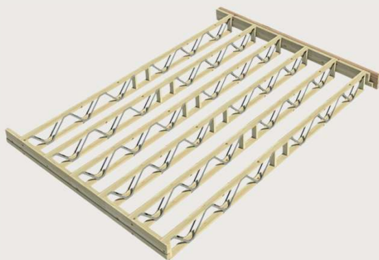
POUTRES POSI
