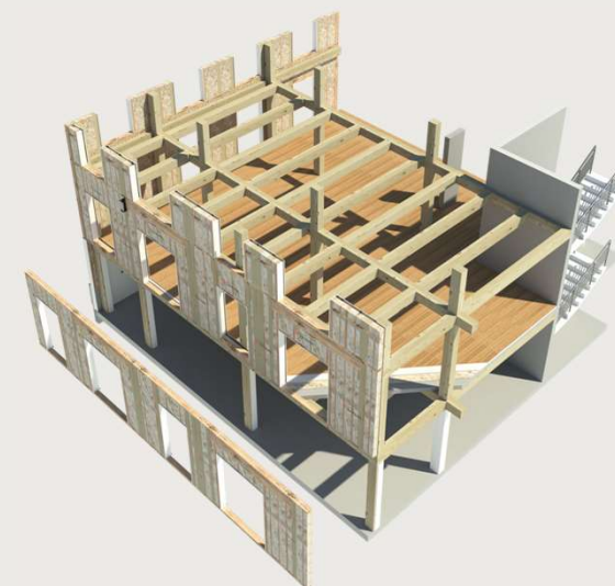
FAÇADES À OSSATURE BOIS Toutes les familles
