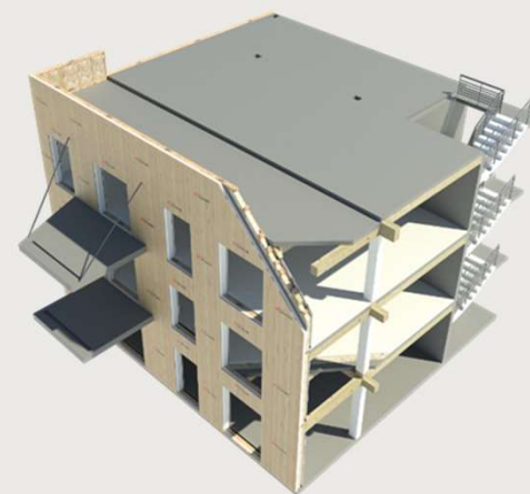
PLANCHERS BOIS BÉTON
